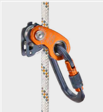
Ascender mode
